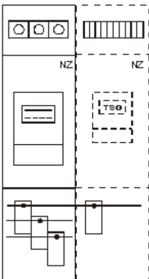
Erweiterung: Sammelschienensystem mit NH-Elementen und Kundenauptsicherung
