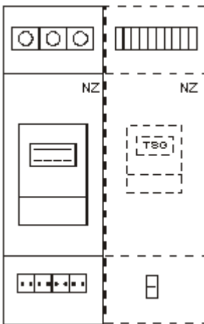
Erweiterung: Anbaukasten mit Klemmstein und Kundenauptsicherung
