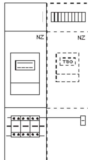
Erweiterung: Sammelschienensystem mit SH-Schalter
