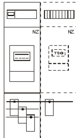
Erweiterung: Sammelschienensystem mit NH-Sicherungen und Kundenauptschalter
