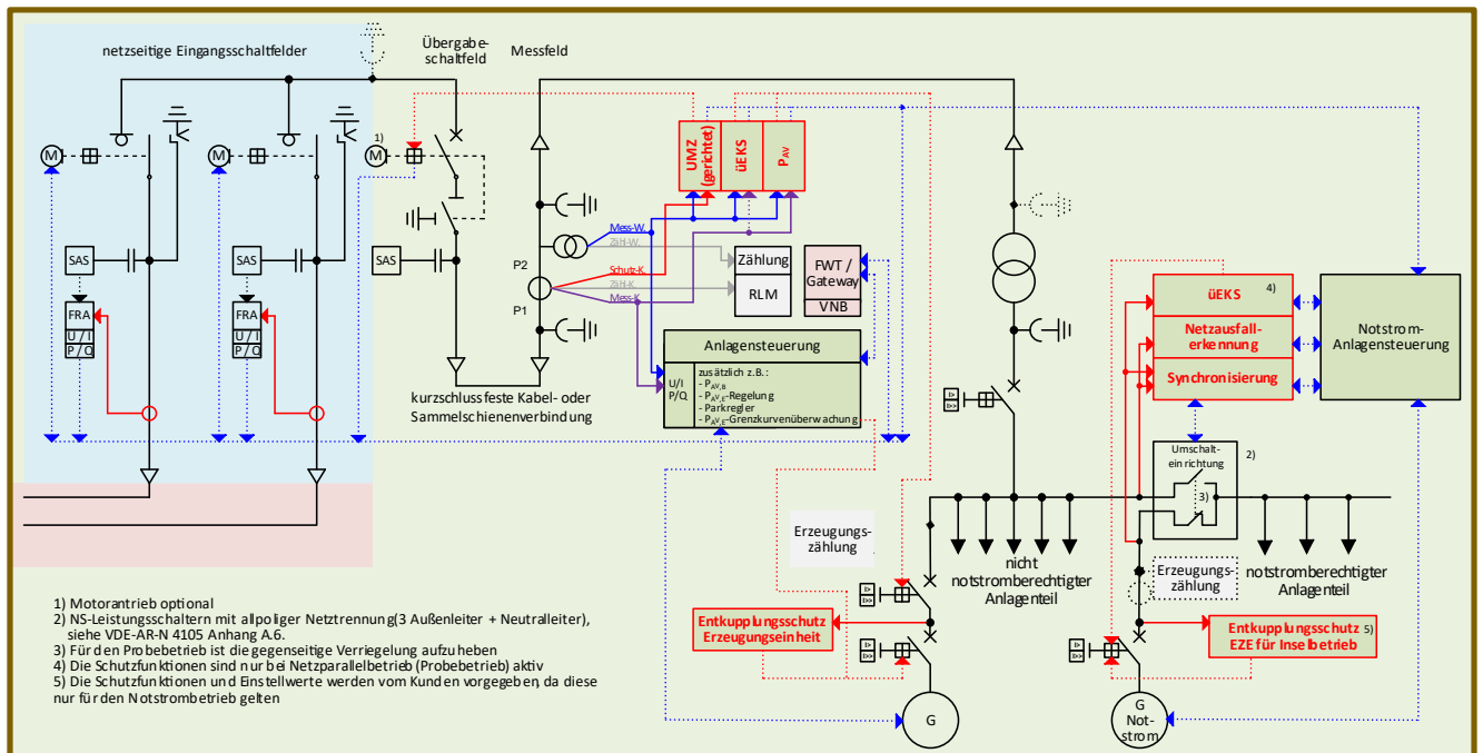
Bild D.9 Ergänzung zu Bild D5 (K)K-TM des BDEW-Musterwortlauts [7]: spezielle Kundenanlagen (K)K-L-M – Notstromanlage mit Probebetrieb parallel zum öffentlichen Netz: MS-Mischanlage – Übergabeschalter als Leistungsschalter , ein Transformator zwei Erzeugungsanlagen, wobei eine als Notstromanlage dient und nur für den monatlich vorgeschriebenen Probebetrieb parallel zum Netz gefahren wird
