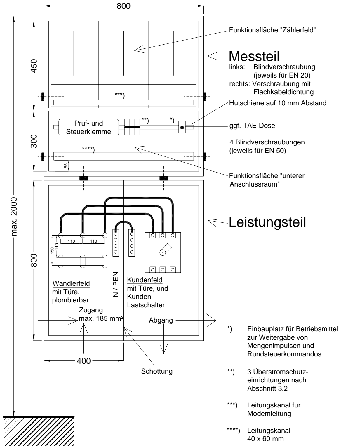
Mess- und Wandlerschrank mit Leistungsteil bis 250 A (halbindirekte Messung)
