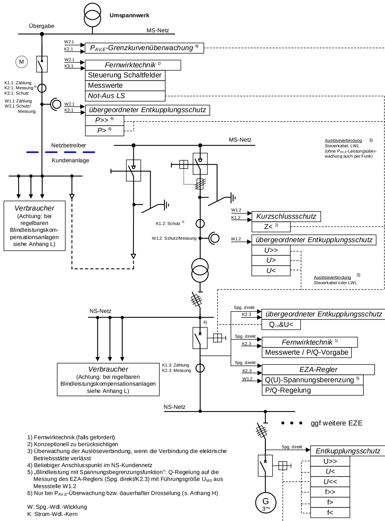
Bild 14-Mischanlage – Beispiel einer an ein Umspannwerk mittelspannungsseitig angeschlossenen Kundenanlage mit Bezug und Erzeugungsanlage mit Lasttrennschalter und einer Erzeugungseinheit ohne Inselbetriebsmöglichkeit
